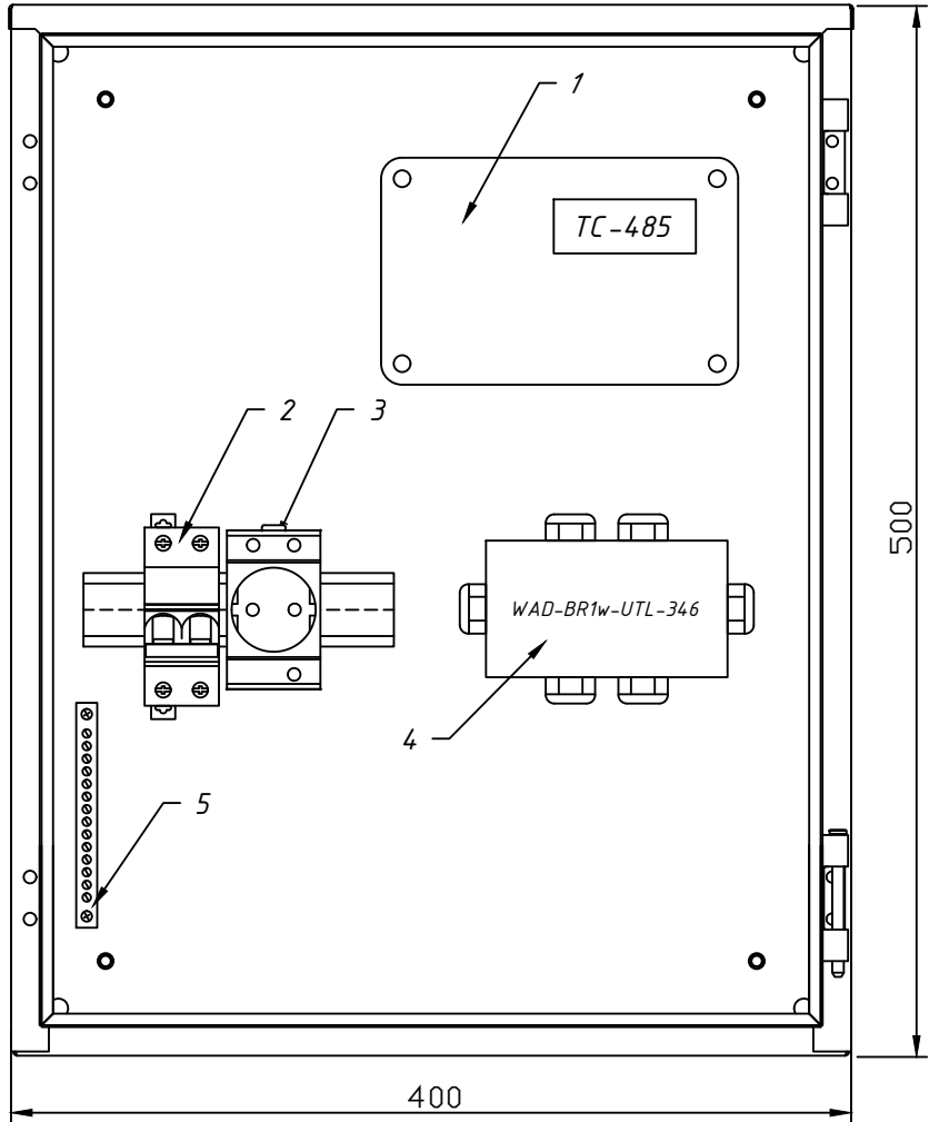
Вид спереду
