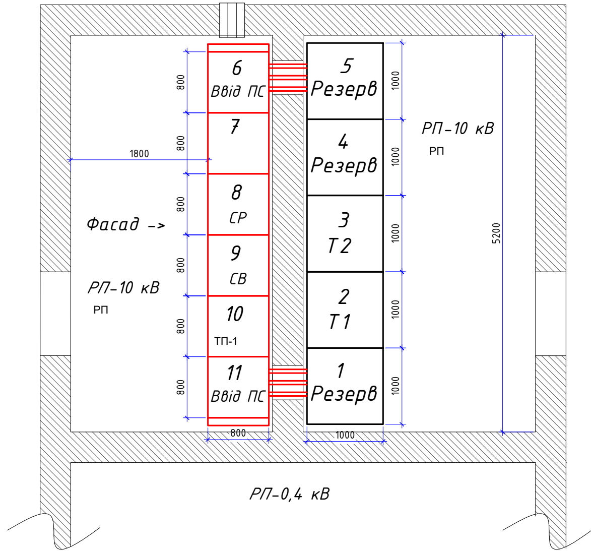
План розташування РП-10 кВ М 1:50
